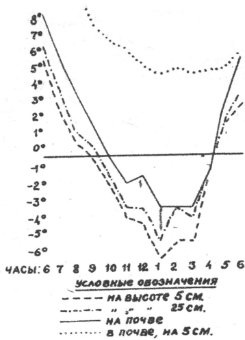
Распределение температуры во время заморозка в ночь с 1/VI на 2/VI 1930 года.
