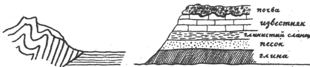
Слои гор и равнин. Расположение слоев на равнине.
